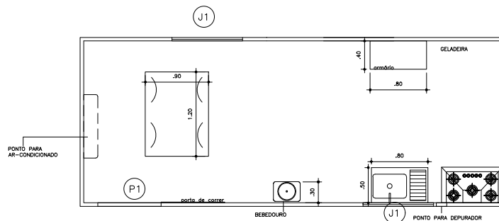
PLANTA BAIXA CONTAINER COZINHA – ITEM 04 Esc. 1:25
