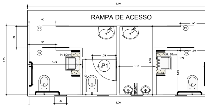
PLANTA BAIXA CONTAINER BANHEIRO – ITEM 02 Esc. 1:25
