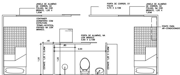
PLANTA BAIXA CONTAINER DORMITÓRIO – ITEM 01 Esc. 1:25
