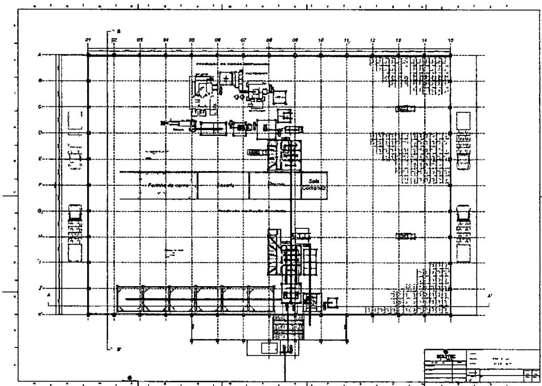
Foto 02 – Planta baixa da fabrica de ração e seus equipamentos.
