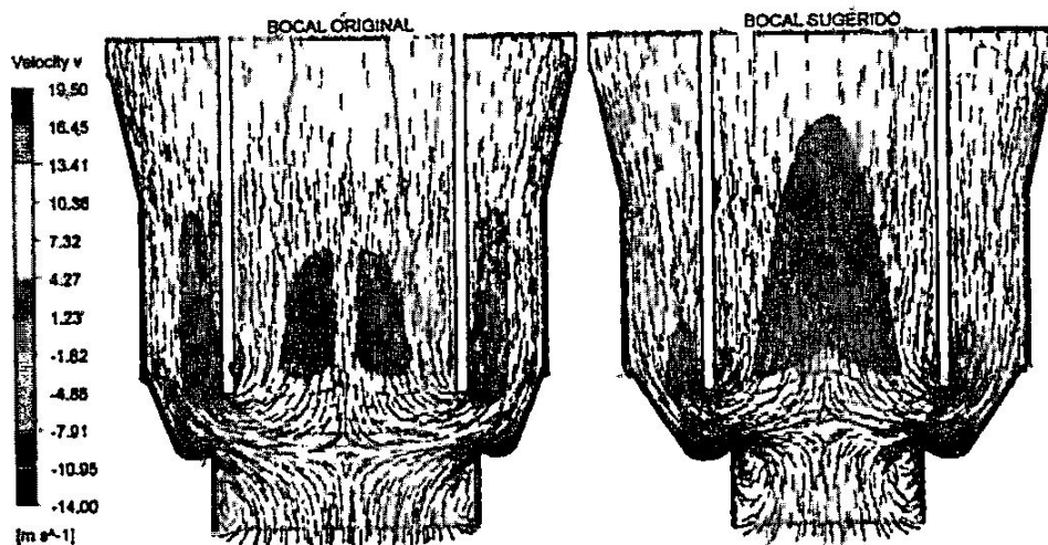
Figura 11 – Campo da componente y da velocidade para o Bocal Original e Bocal Sugerido em um plano central ao calador na região do bocal com vetores indicando o sentido do escoamento.
