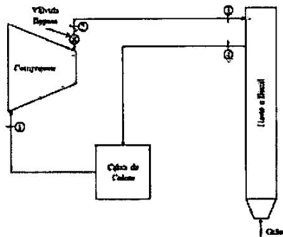
Figura 9 – Fluxograma esquemático do equipamento em estudo.
