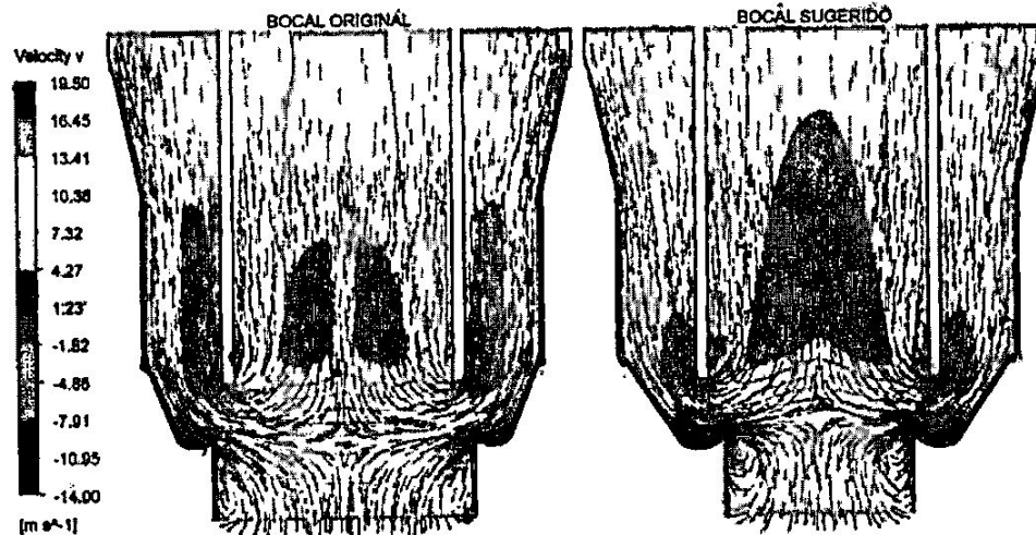
Figura 11 – Campo da componente y da velocidade para o Bocal Original e Bocal Sugerido em um plano central ao eixo na região do bocal com vetores indicando o sentido do escoamento.
