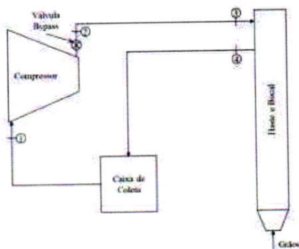
Figura 9 – Fluxograma esquemático do equipamento em estudo.
