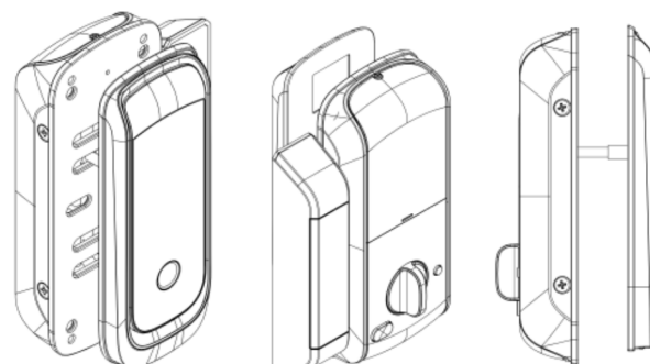
Unidade Exterior
