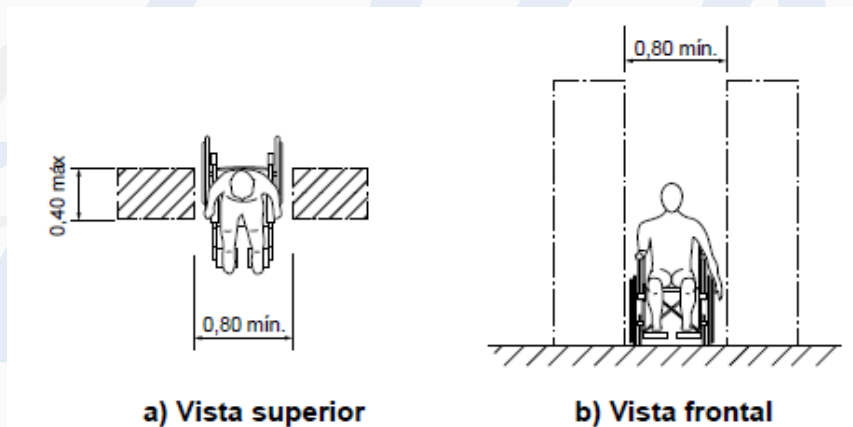
Figura 5 da ABNT NBR 9050: 2015 – Transposição de obstáculos isolados
