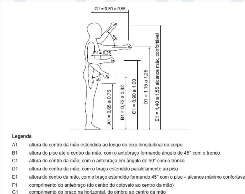
Figura 11 da ABNT NBR 9050: 2015 – Alcance manual frontal – Pessoa em pé
