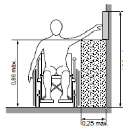
Figura 14 da ABNT NBR 9050: 2015 – Alcance manual lateral sem deslocamento do tronco
