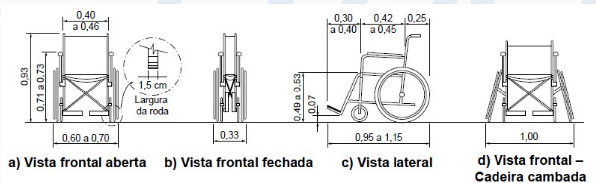
Figura 2 da ABNT NBR 9050:2015 – Cadeira de rodas manual, motorizada e esportiva.
