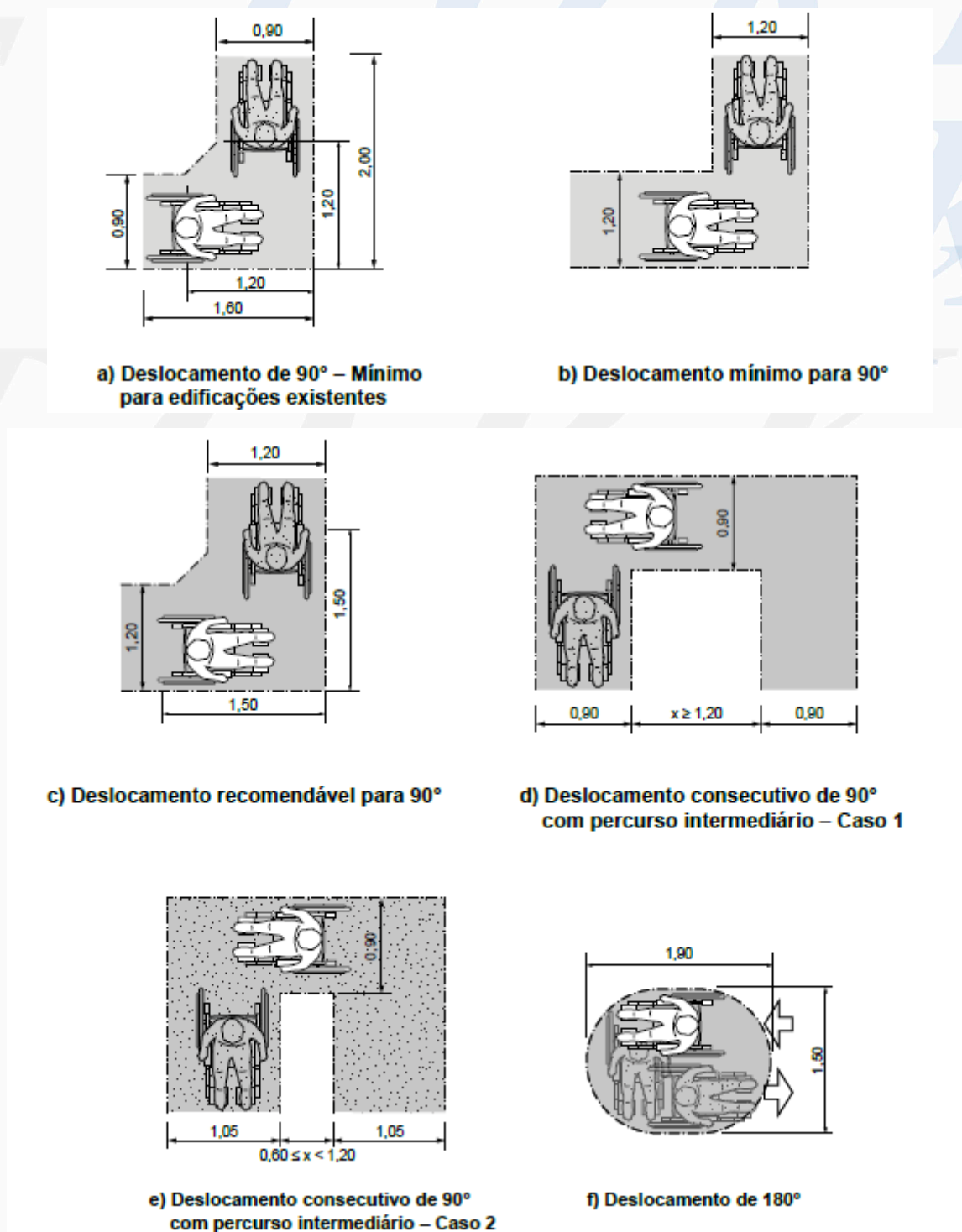
Figura 8 da ABNT NBR 9050: 2015 – Área para manobra de cadeiras de rodas com deslocamento
