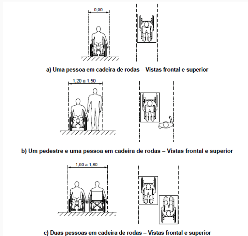
Figura 4 da ABNT NBR9050: 2015 – Largura para deslocamento em linha reta
