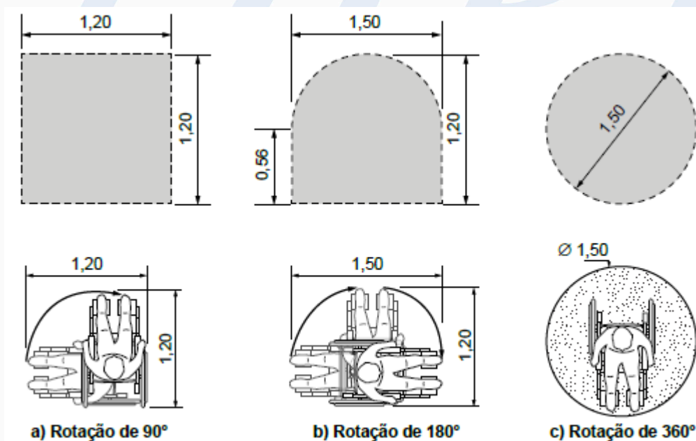
Figura 7 da ABNT NBR 9050: 2015 – Área para manobra de cadeira de rodas sem deslocamento
