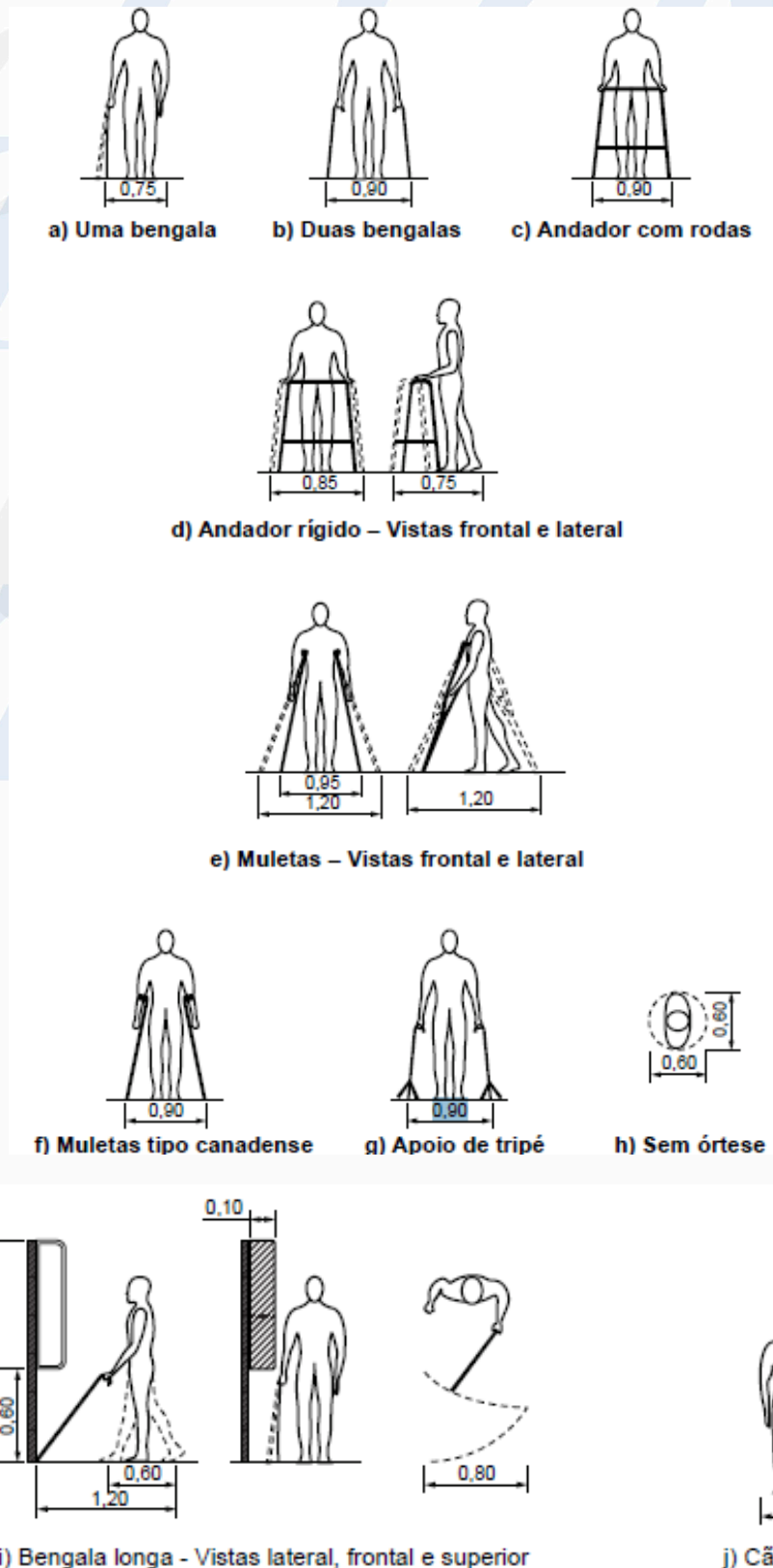
Figura 1 da ABNT NBR 9050:2015 – Dimensões referenciais para descolamento de pessoa em pé.
