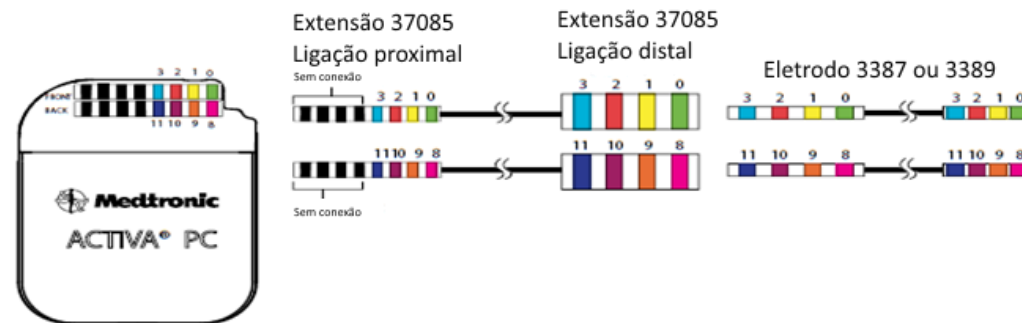
Diagrama de conexões do Activa PC e Activa RC com adaptador
