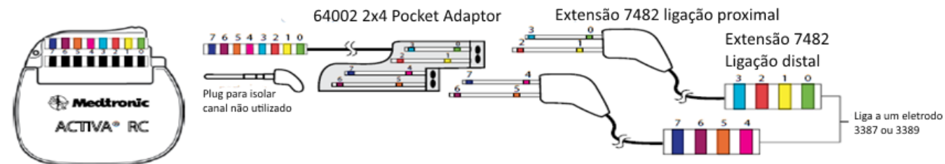
Diagrama de conexões do Activa PC e Activa RC com adaptador
