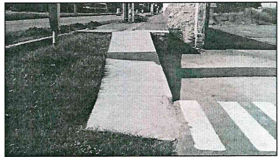
Figura 22 - Construção da rampa e instalação de condutores de águas pluviais
