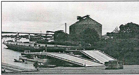
Figura 21- rampas flutuantes
