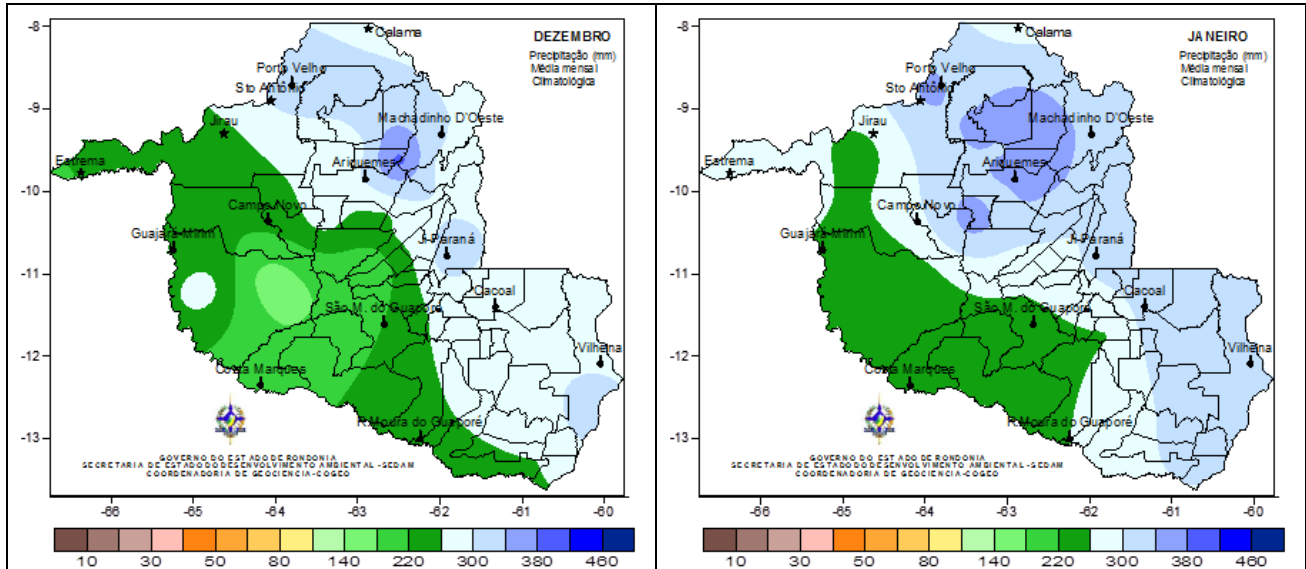
Fig. A- Climatologia de precipitação mensal, baseada nos métodos dos Quantis - 1970 a 2011.
