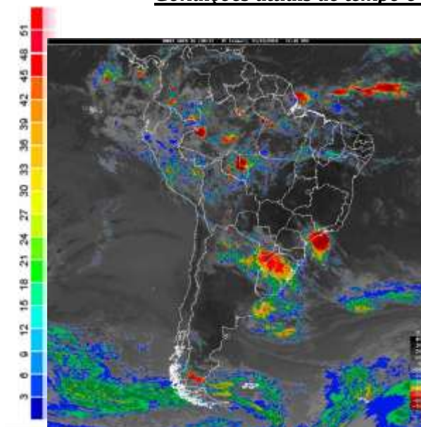
Fig. 1- Mapa da precipitação de 21/12/2018: Imagem Góes 13 canal infravermelho.
