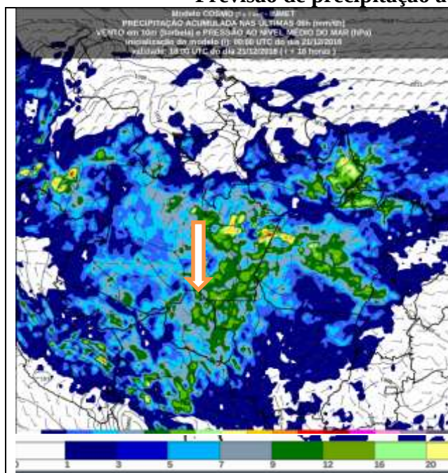
FIGURA 2 – Previsão do tempo no Estado de Rondônia para o dia 21/12/2018 as 18UTC
