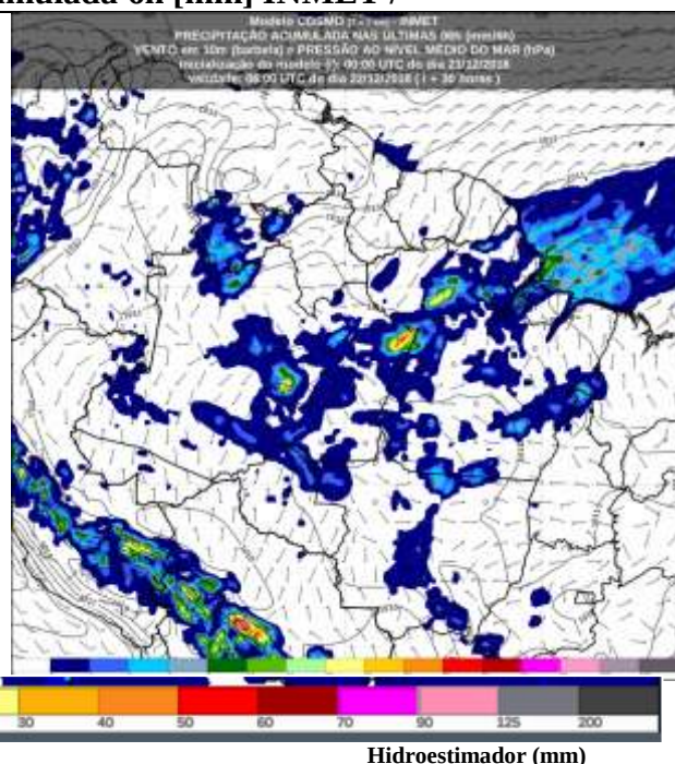
Fig. 3 – Previsão do tempo no Estado de Rondônia para o dia 22/12/2018 as 06 UTC
