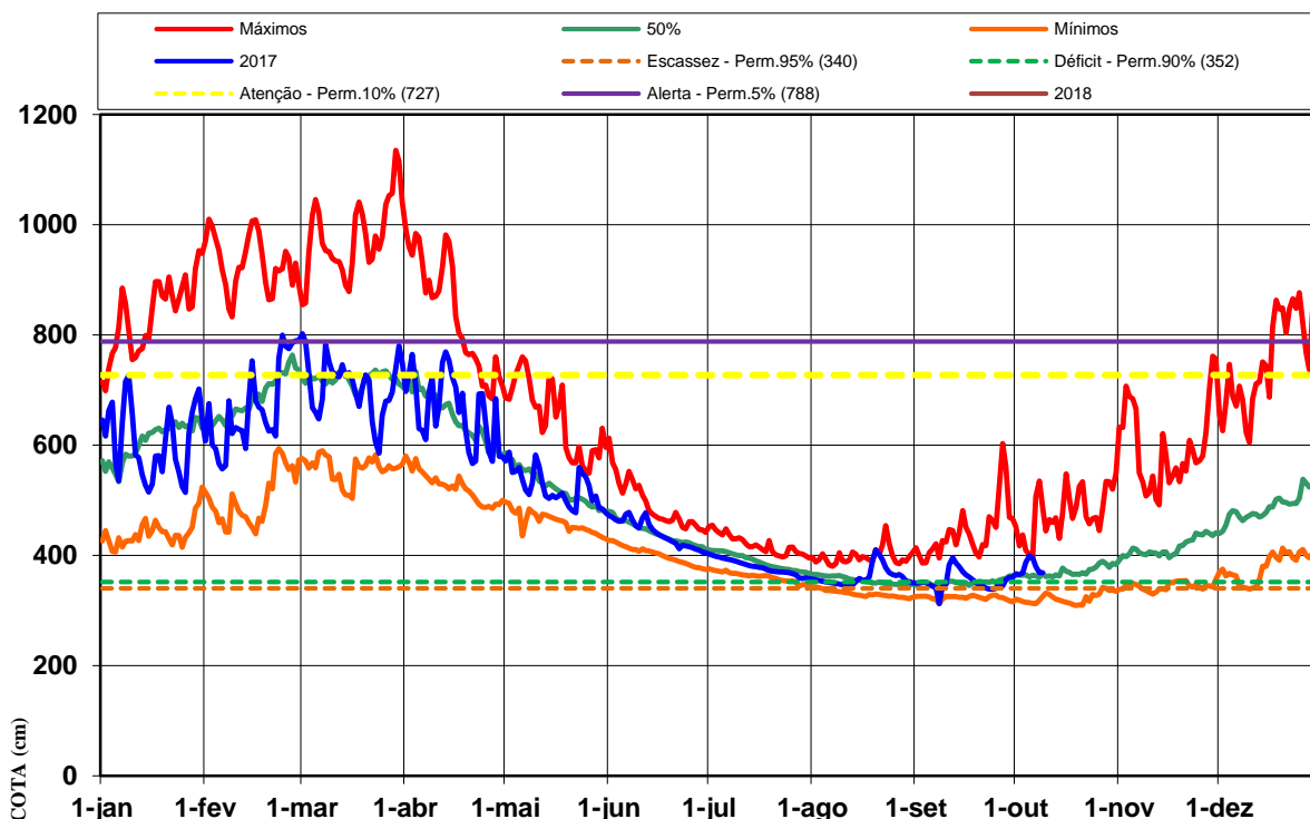
Gráfico - Monitoramento diário da cota do rio Jaru, série histórica 1978 – 2017, na coordenada geográfica de latitude 10,4458° leste e longitude 62,4256° oeste, Ponte Br-364, Jaru/RO.
