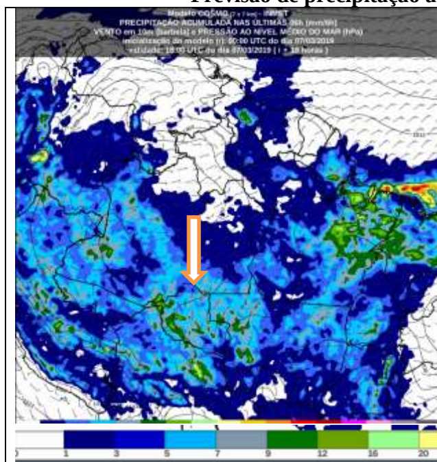
FIGURA 2 – Previsão do tempo no Estado de Rondônia para o dia 07/03/2019 às 18UTC
