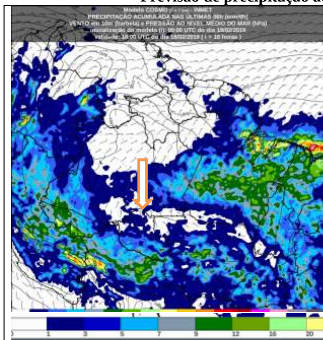
FIGURA 2 – Previsão do tempo no Estado de Rondônia para o dia 18/02/2019 as 18UTC
