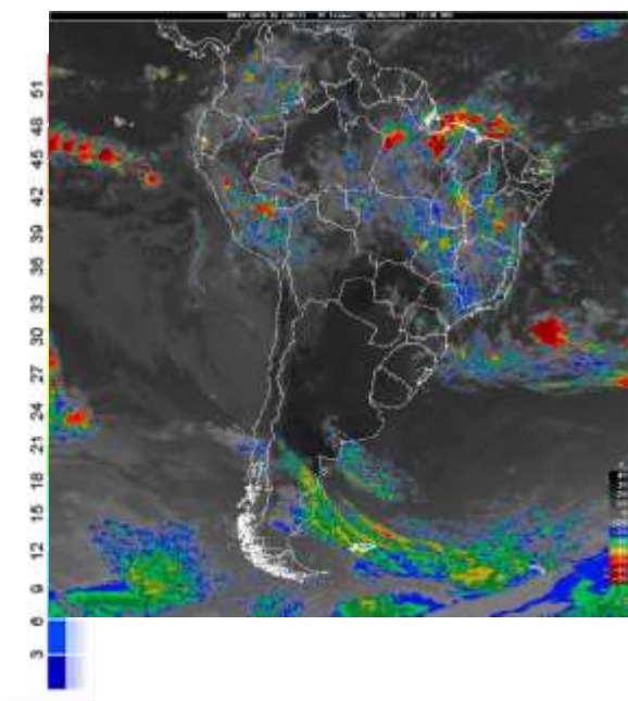
Fig. 1- Mapa da precipitação de 18/02/2019: Imagem Góes 13 canal infravermelho.
