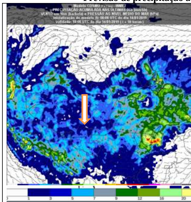
FIGURA 2 – Previsão do tempo no Estado de Rondônia para o dia 14/01/2019 às 18UTC
