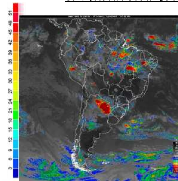
Fig. 1- Mapa da precipitação de 14/01/2019: Imagem Góes 13 canal infravermelho.
