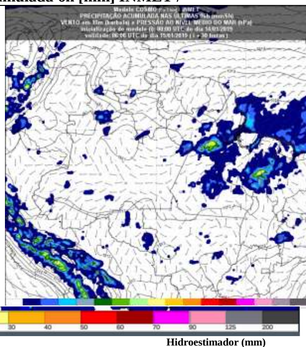
Fig. 3 – Previsão do tempo no Estado de Rondônia para o dia 15/01/2019 às 06 UTC
