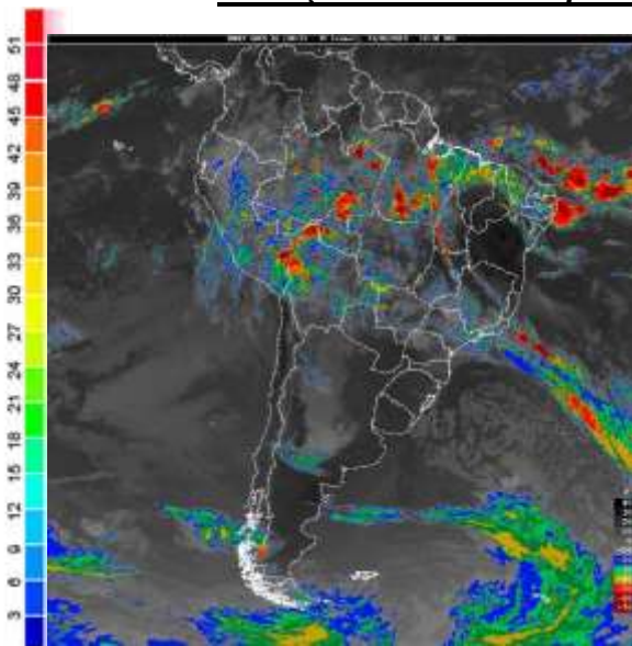
Fig. 1- Mapa da precipitação de 13/02/2019: Imagem Góes 13 canal infravermelho.
