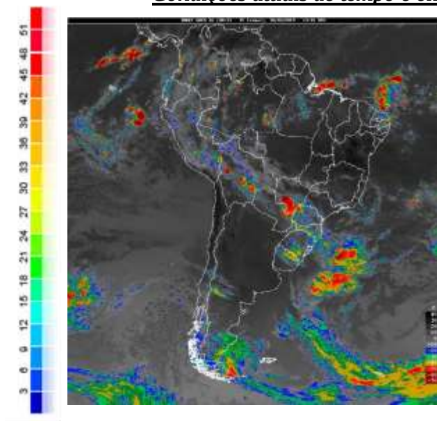
Fig. 1- Mapa da precipitação de 18/03/2019: Imagem Góes 13 canal infravermelho.
