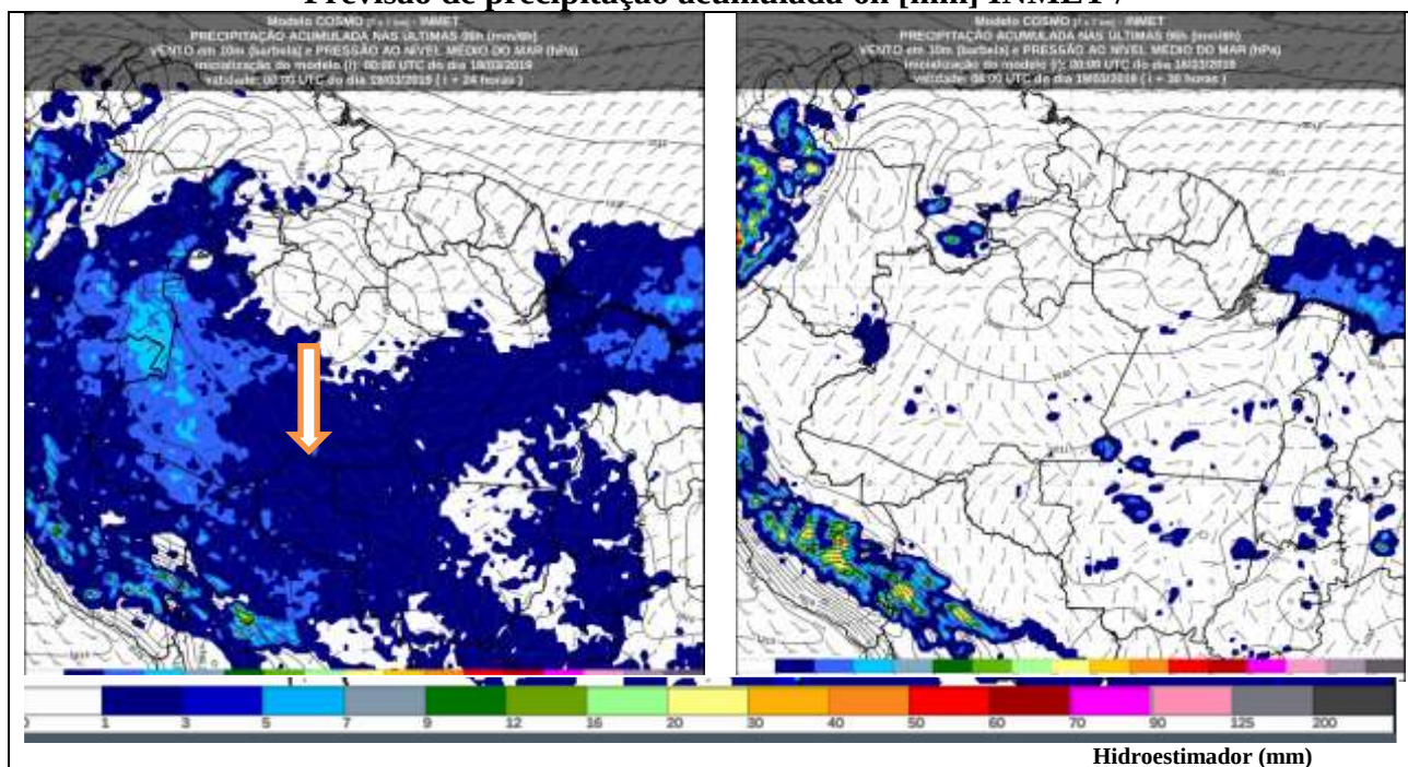
FIGURA 2 – Previsão do tempo no Estado de Rondônia para o dia 18/03/2019 às 18UTC
